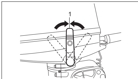
1. Pozycja „NEUTRAL”
