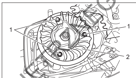
1. Śruba 2. Wentylator
