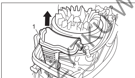
1. Kanał powietrzny
