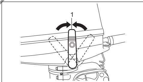
1. Pozycja „NEUTRAL”
