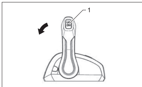
1. Górna część przycisku PTT
