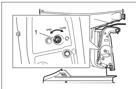
1. Śruba ręcznego zwalniania (DF300B, DF325A, DF350A)
