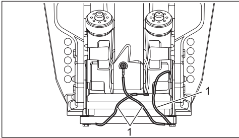
1. Przewód uziemiający (DF300B, DF325A, DF350A)
