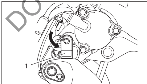
1. Wspornik pochylenia (DF300BMD, DF350AMD)
