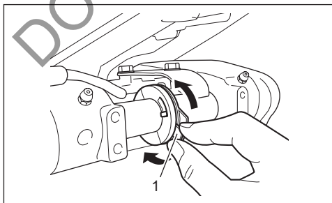
1. Uchwyt
