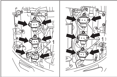
1. Uchwyt cewki zapłonowej
