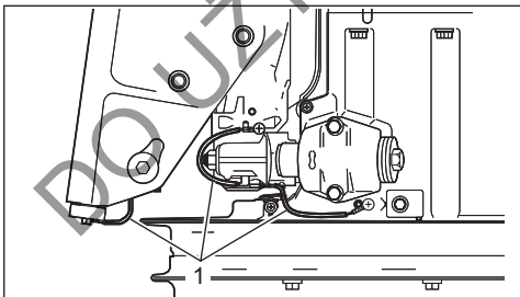
1. Przewód uziemiający (DF300BMD, DF350AMD)
