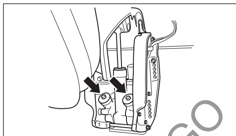
1. Śruba ręcznego zwalniania (DF300BMD, DF350AMD)
