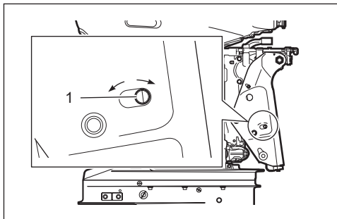
1. Śruba ręcznego zwalniania (DF300BMD, DF350AMD)
