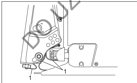
1. Przewód uziemiający (DF70AT, DF75RT, DF80AT, DF90AT, DF100BT)
