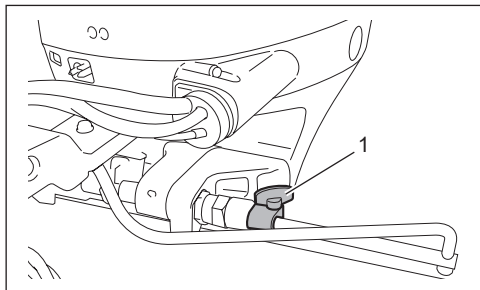
1. Śruba regulacyjna oporu sterowania
