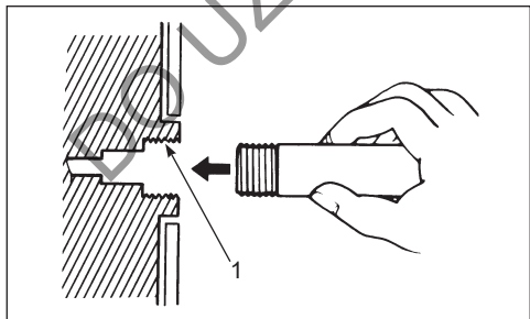
1. Gwint kanału do przepłukiwania
